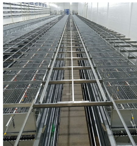
Модернизация птицеводческого комплекса АО «Птицефабрика Роскар»
