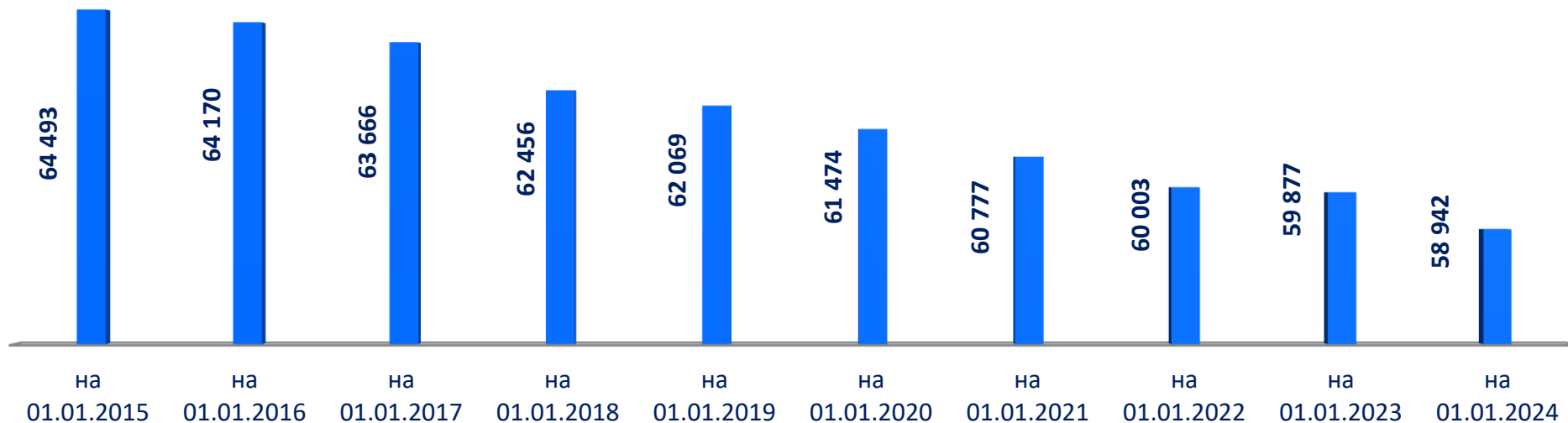
График 2
